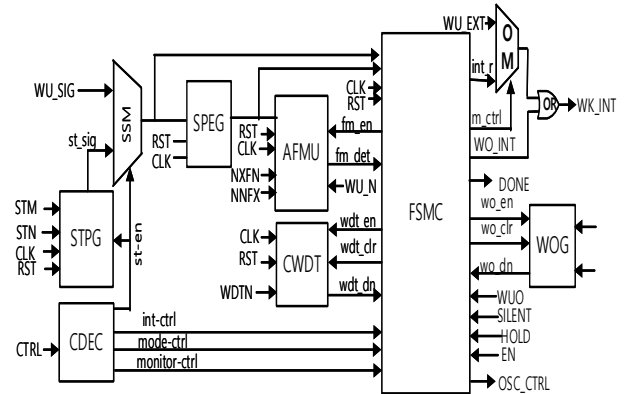
Fig. 5. RF WuRx intelligent digital controller (IDC) architecture
