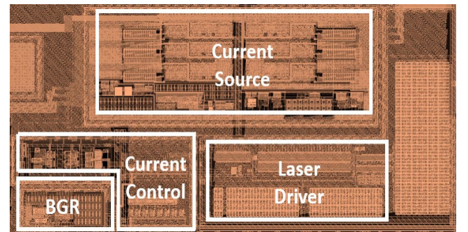
Fig. 15. FDNIRS TX floorplan
