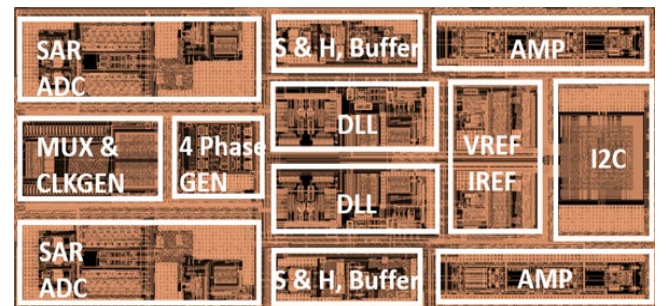
Fig. 16. FDNIRS RX floorplan
